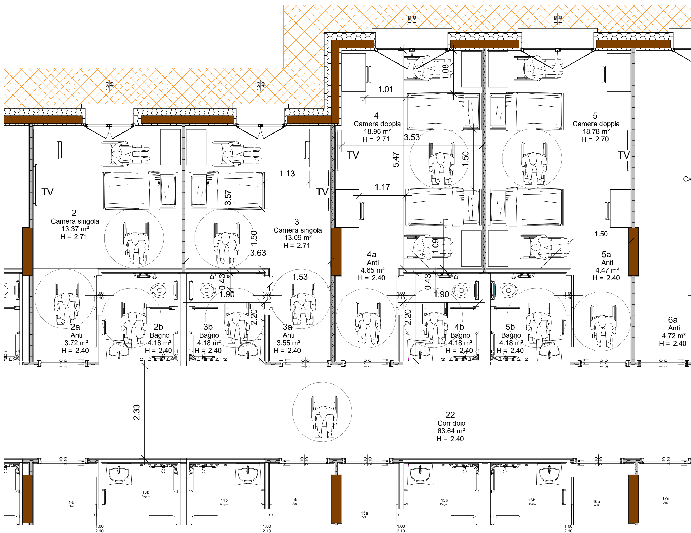
Particolare Camere tipo - Scala 1:50
